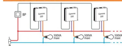
REPRÉSENTATION DE LA PUISSANCE SUR UN CIRCUIT RING (LA SERIE 500)
