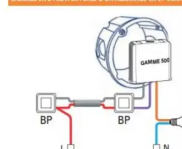
CÂBLAGE EN 2 FILS À LA PLACÉ D'UN ALLUMAGE VA-ET-VIENT
