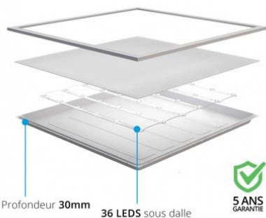
36 LEDS sous dalle
