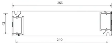
Dimensions en mm de profil
